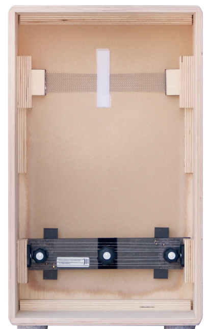
Abbildung zeigt Innenleben von CP580
